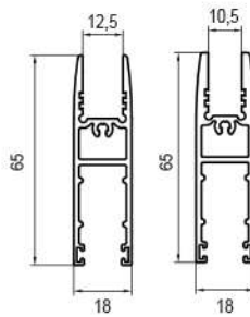
Perfil marco lateral
