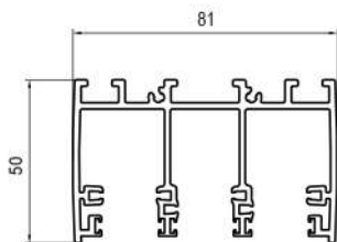
Perfil guía superior T3
