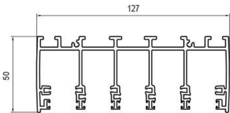
Perfil guía superior T5
