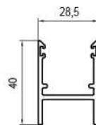
Perfil de hoja
